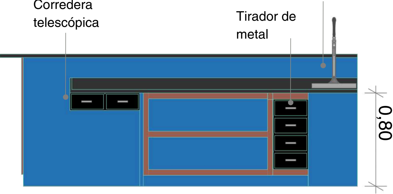
Vista: Frente.
