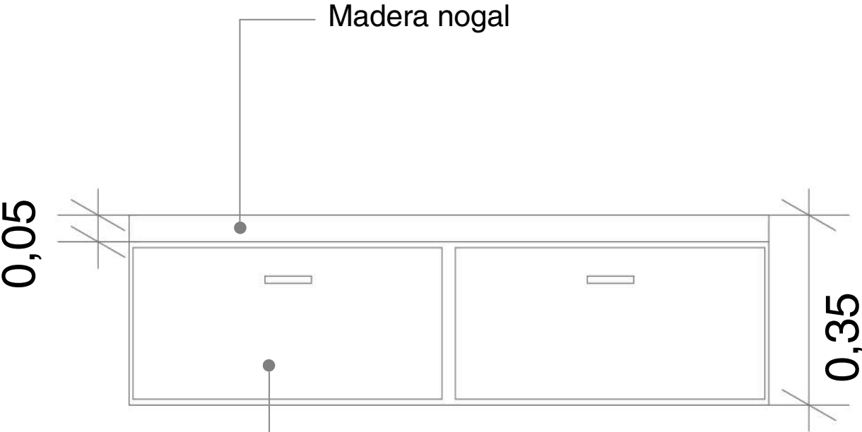
Vista: frente.
