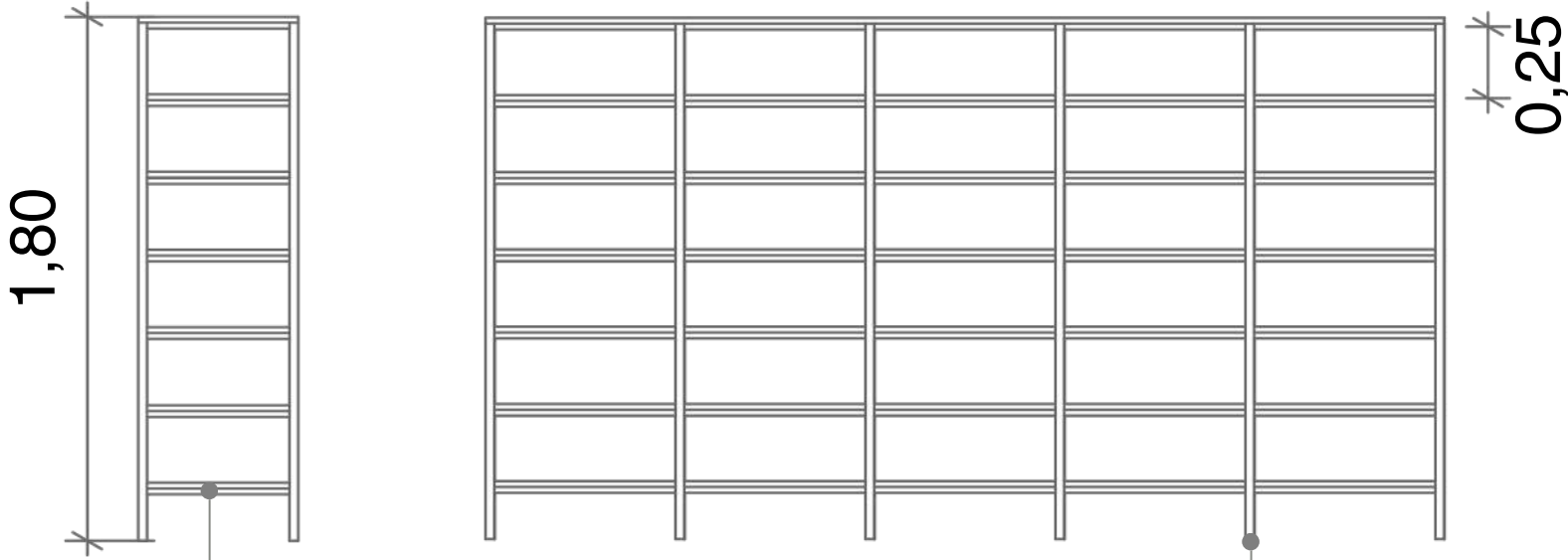
Vista: costado.
