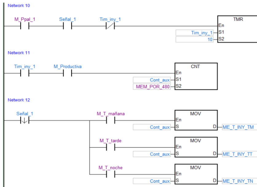
Figura 9: Circuito (Fuente: Trabajo Final Romero)
