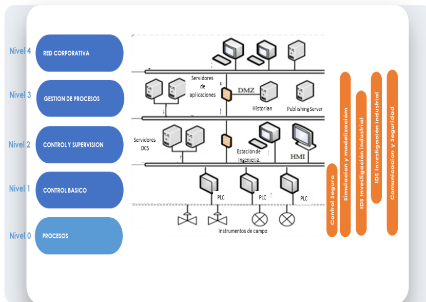
Figura 6: Arquitectura de SCI ajustada a modelo ISA-95 (Fuente: INCIBE)
