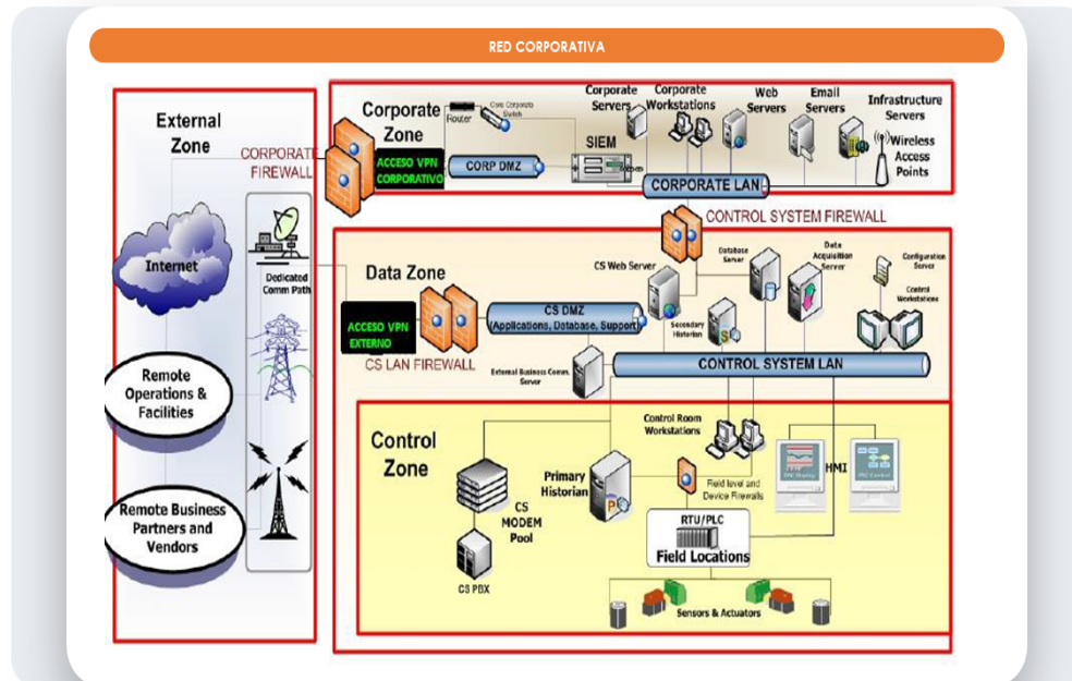
Figura 7: Arquitectura de SCI ajustada a modelo pirámide ISA (Fuente: INCIBE)
