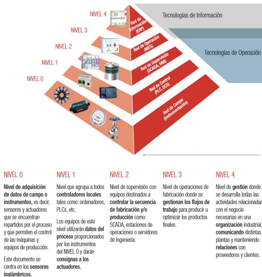
Figura 3: Niveles Purdue (Fuente: Centro de Ciberseguridad Industrial - CCI) 1
