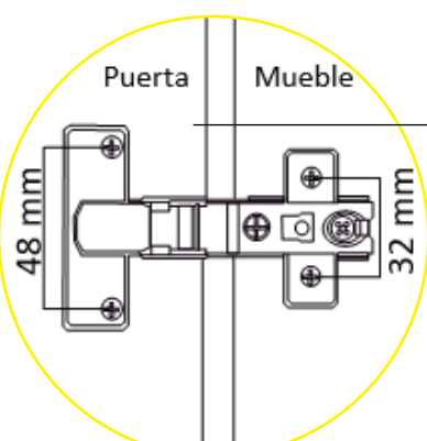
Unión mueble con puerta
