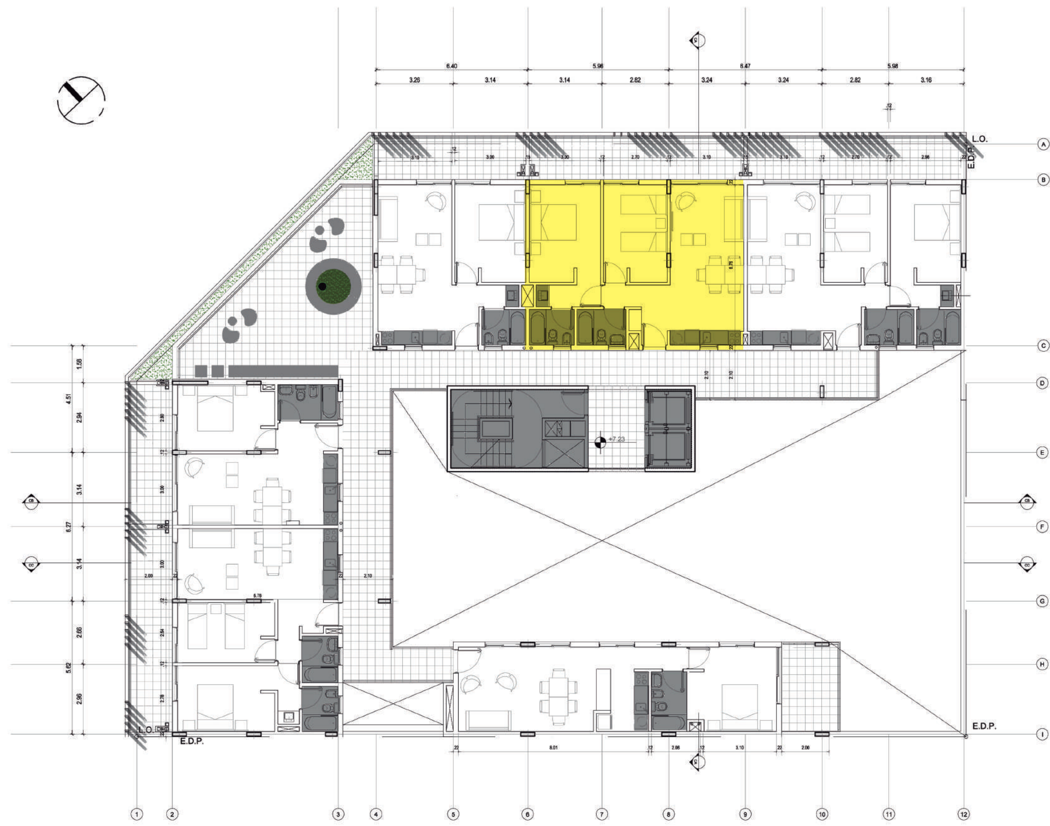
PLANTA 3º TERRAZA NIVEL +10,05
